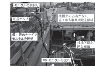
国土交通大臣賞 圧入施工が可能な超高耐久性モルタル による補修技術(スリムフローグラ ウト工法)の開発 株式会社大林組
