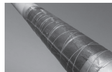
経済産業大臣賞 送電用鋼管鉄塔の部材腐食に伴う現 場VaRTM工法によるCFRP補修技 術の開発 東京電力パワーグリッド株式会社
